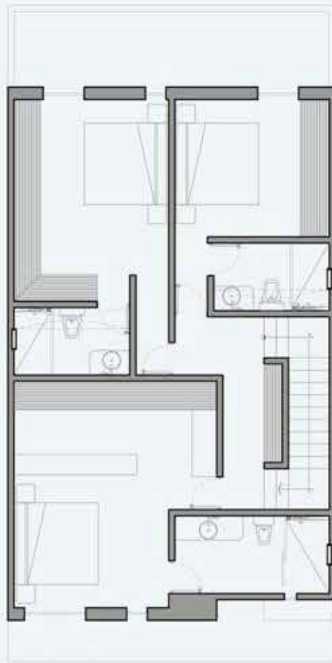
PLANTA ALTA
